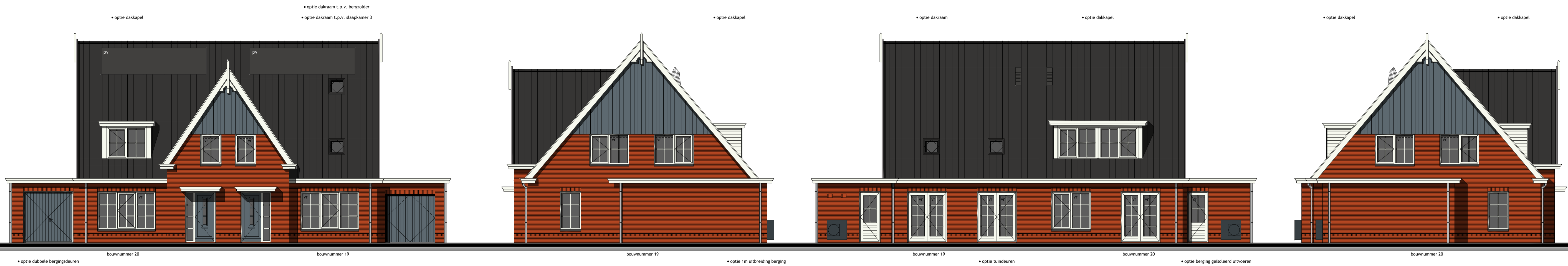
Voorgevel
