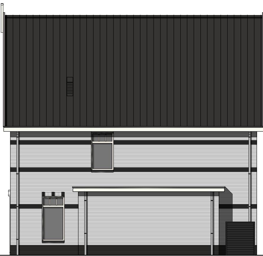
Rechter zijgevel
